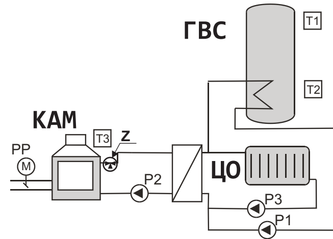
Рис.16 Схема работы регулятора с теплообменником для ЦО (насос теплообменника и насос ЦО подключенные на выходе P3)
